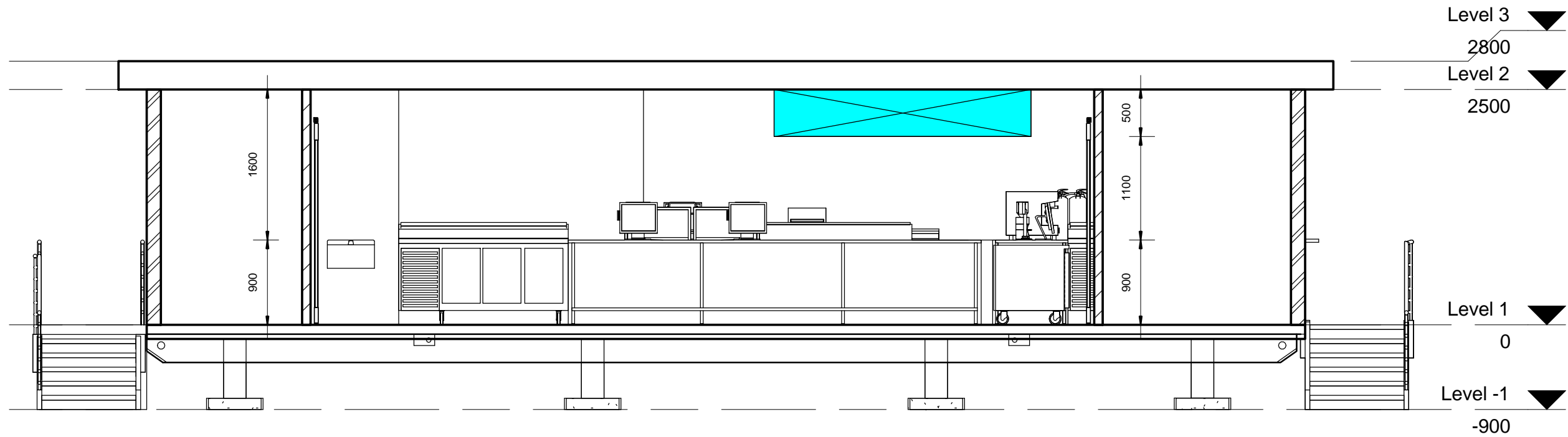
1 Section 7 1 : 50
