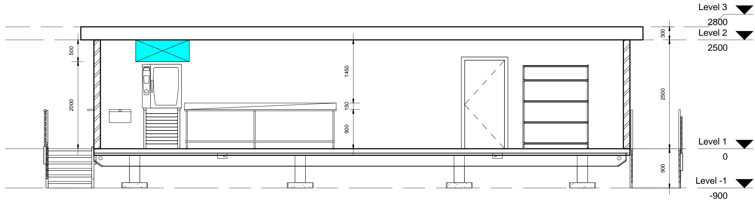
1 Section 1 1 : 50
