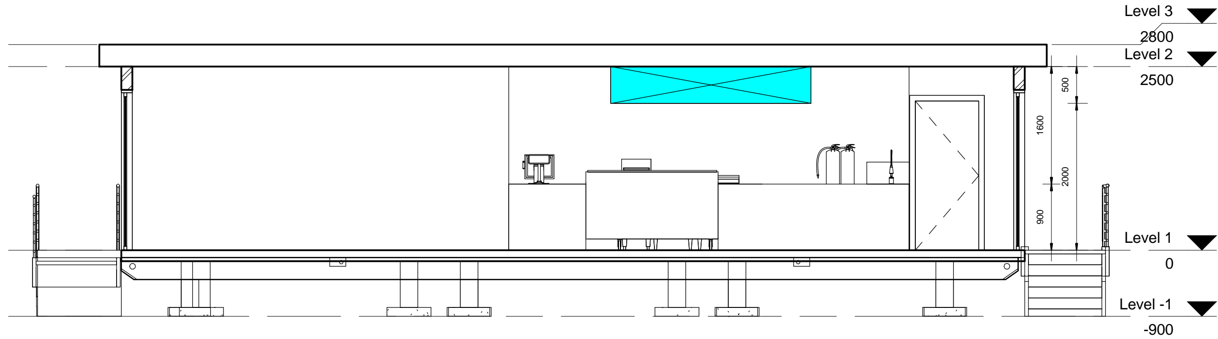
1 Section 5 1 : 50
