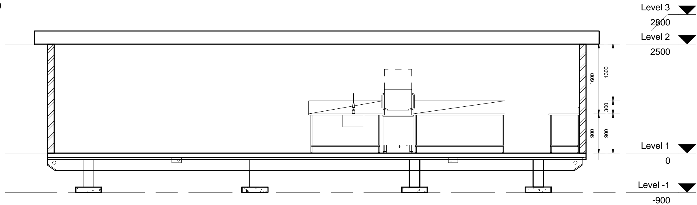
2 Section 2 1 : 50
