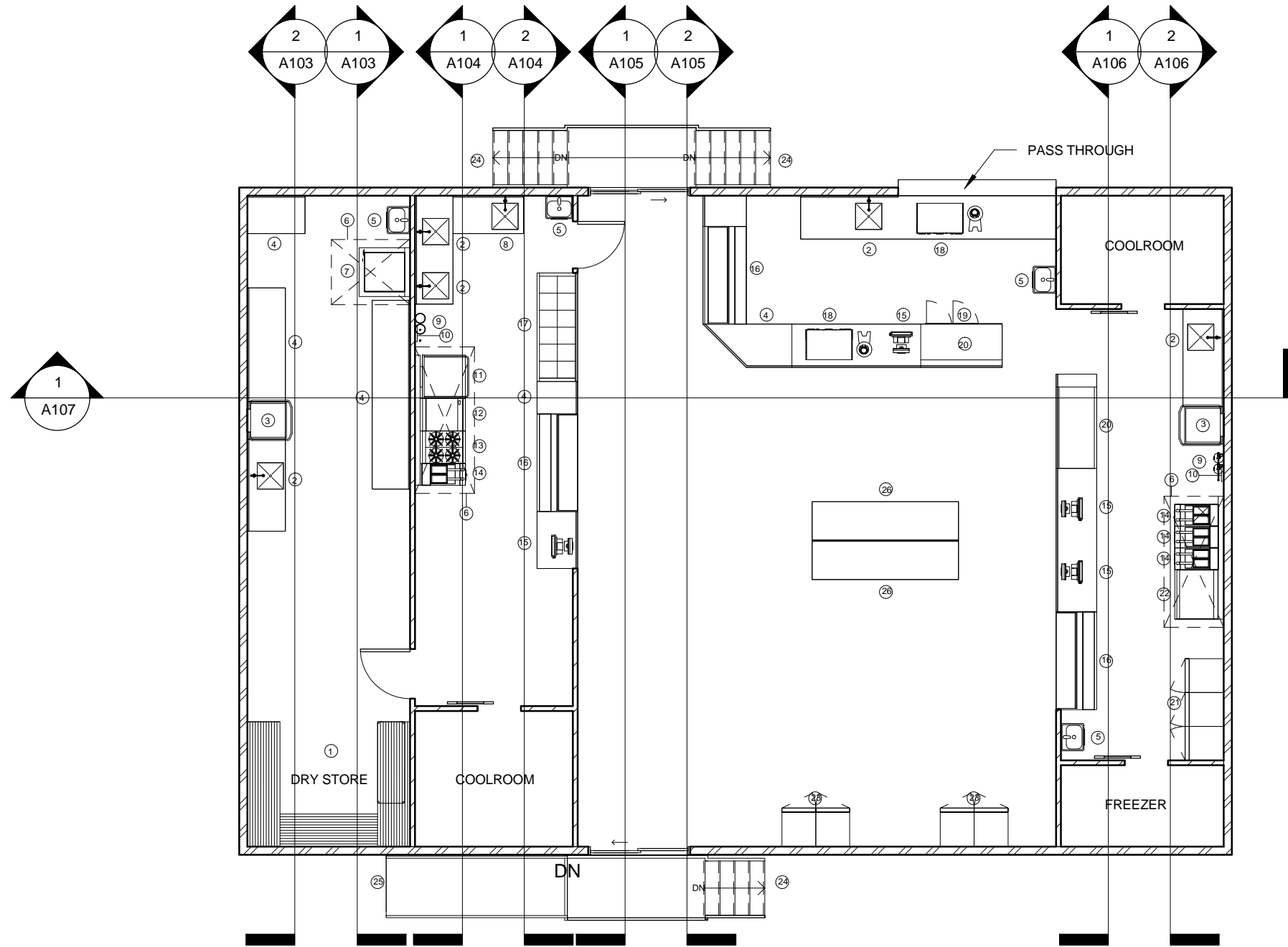
1 Section Cut Plan 1 : 100
