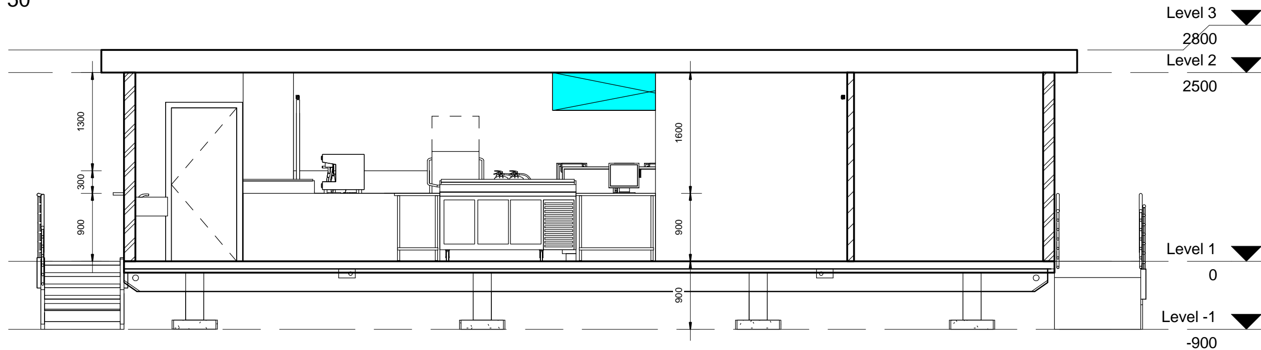
2 Section 4 1 : 50
