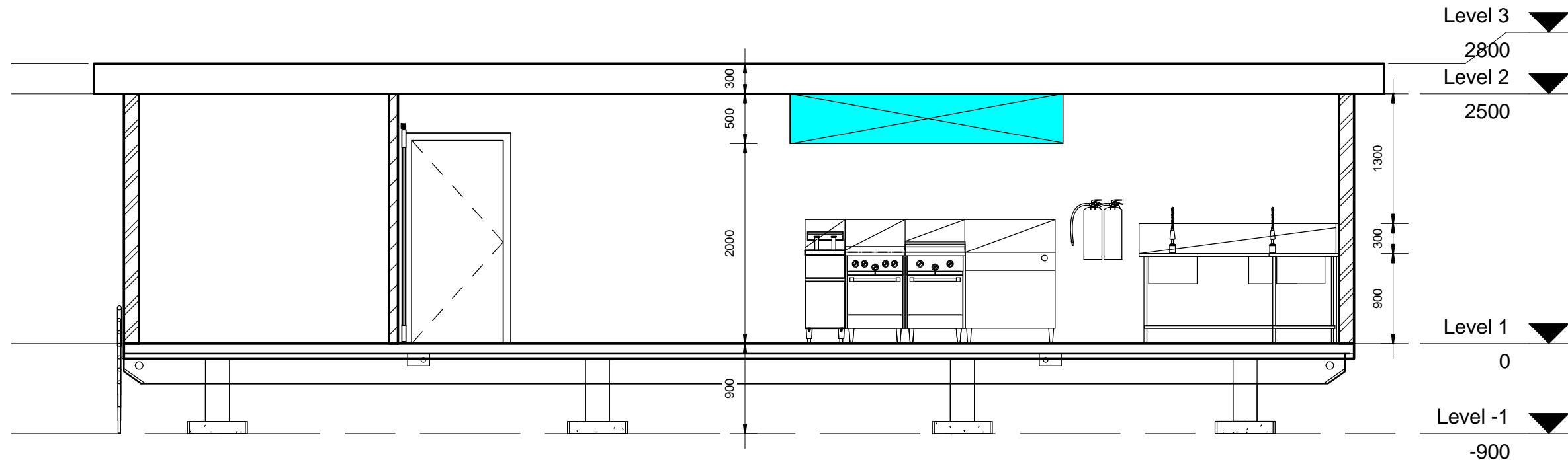
1 Section 3 1 : 50
