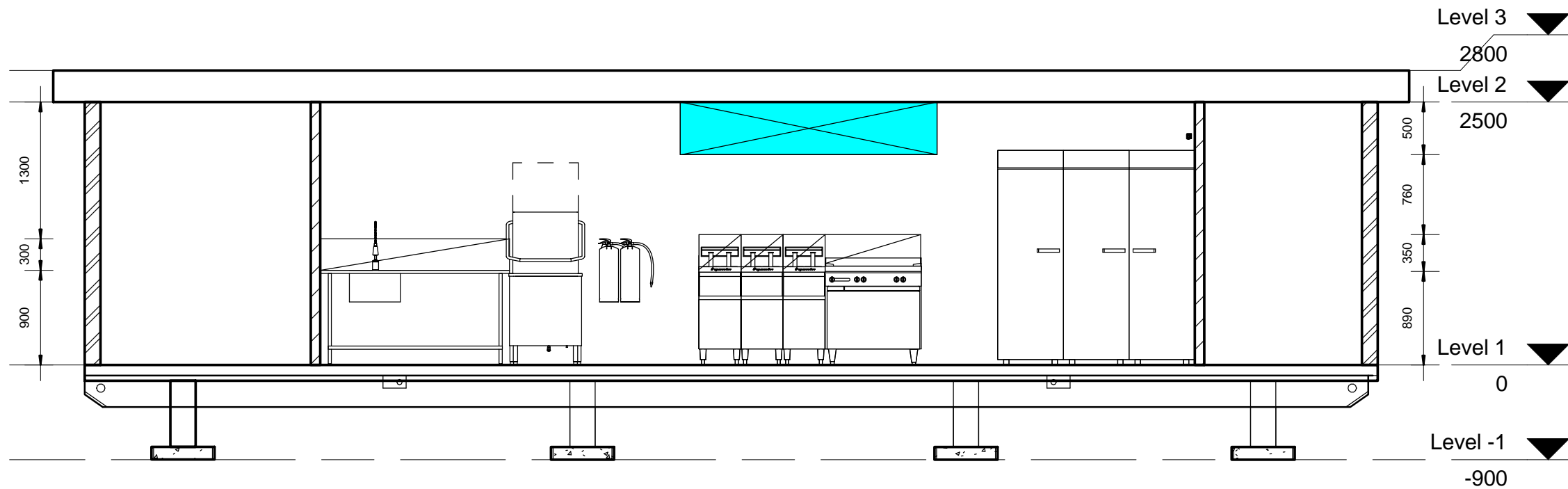
2 Section 8 1 : 50
