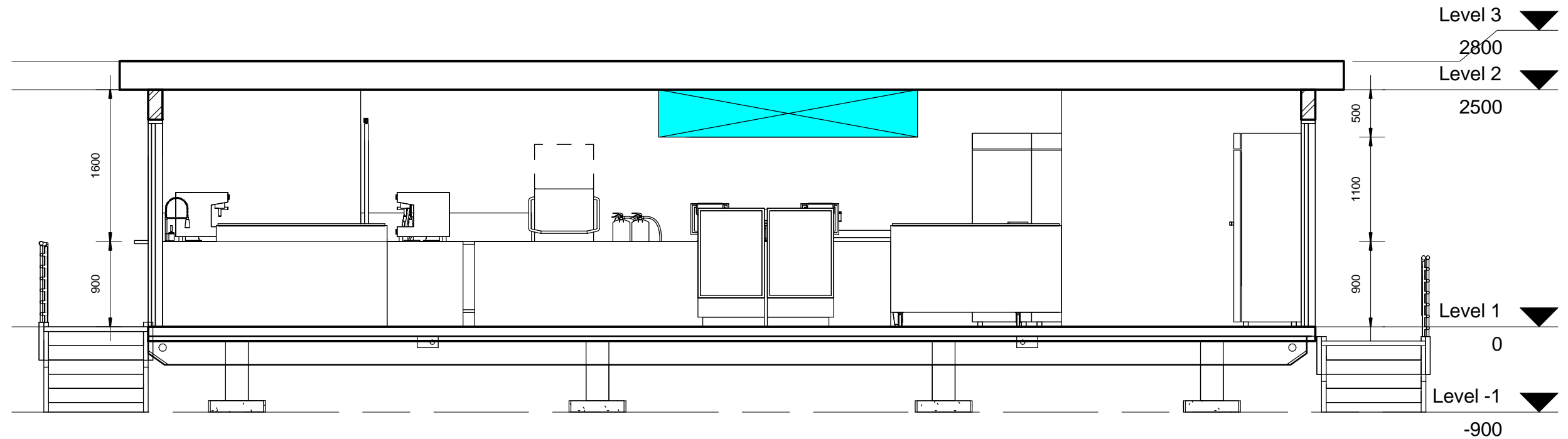
2 Section 6 1 : 50
