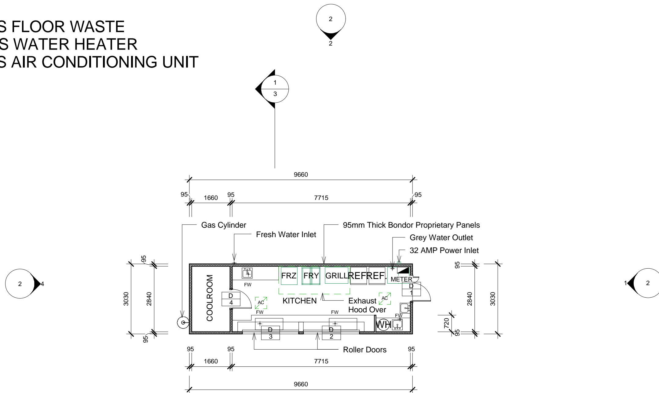
1 Floor Plan 1 : 100
